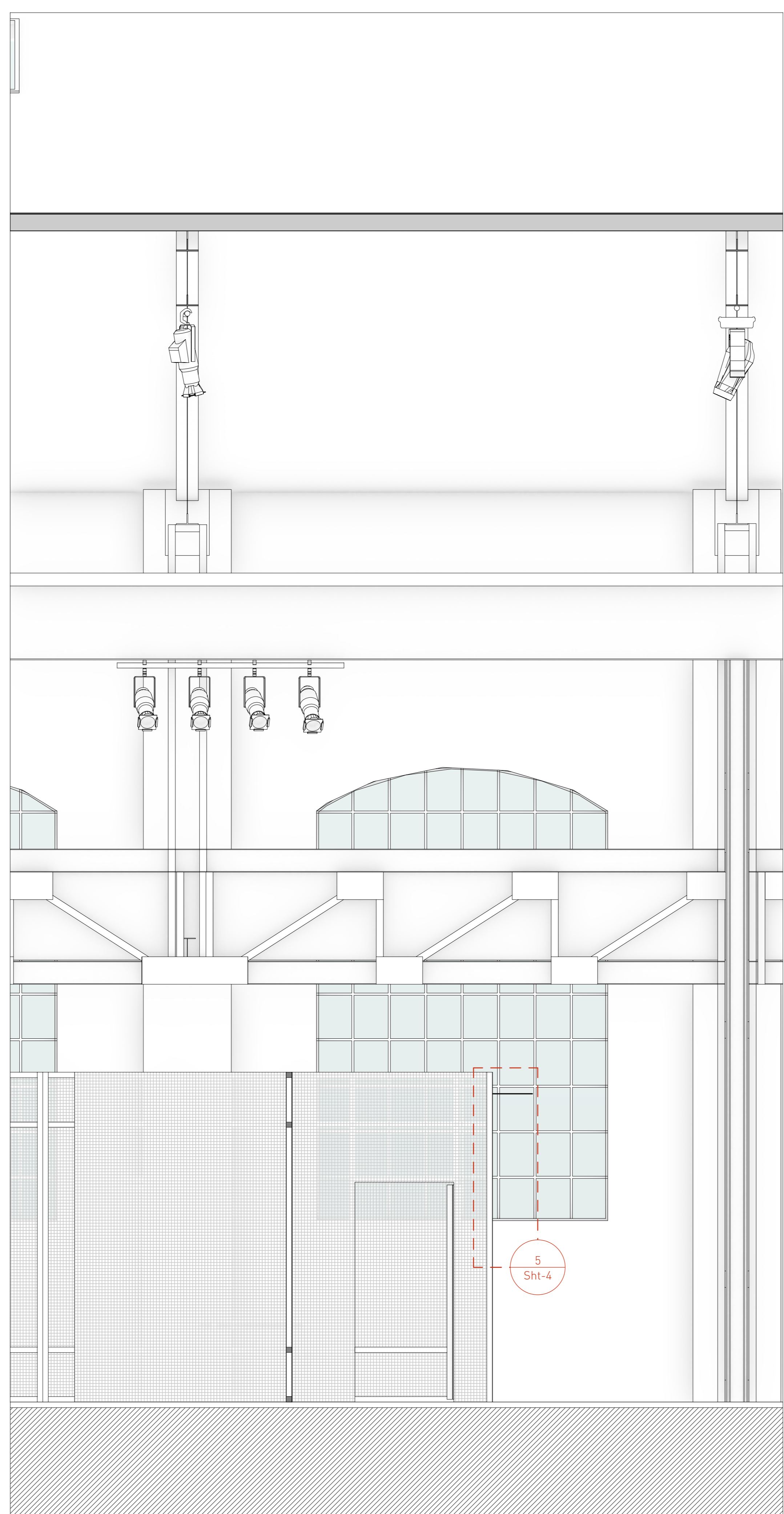
2 WEST FACING Scale: 1:25
